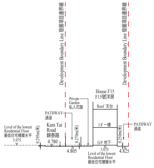
橫截面圖 N-N CROSS-SECTION PLAN N-N
