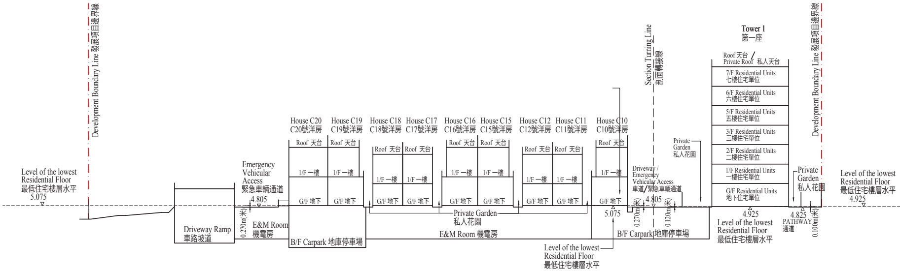
橫截面圖 J-J CROSS-SECTION PLAN J-J
