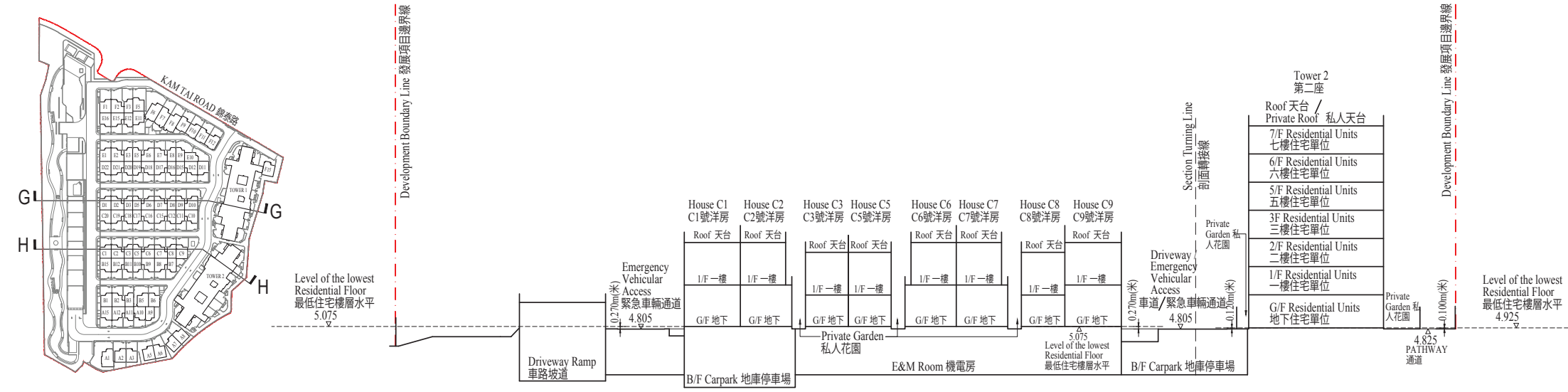
橫截面圖 G-G CROSS-SECTION PLAN G-G
