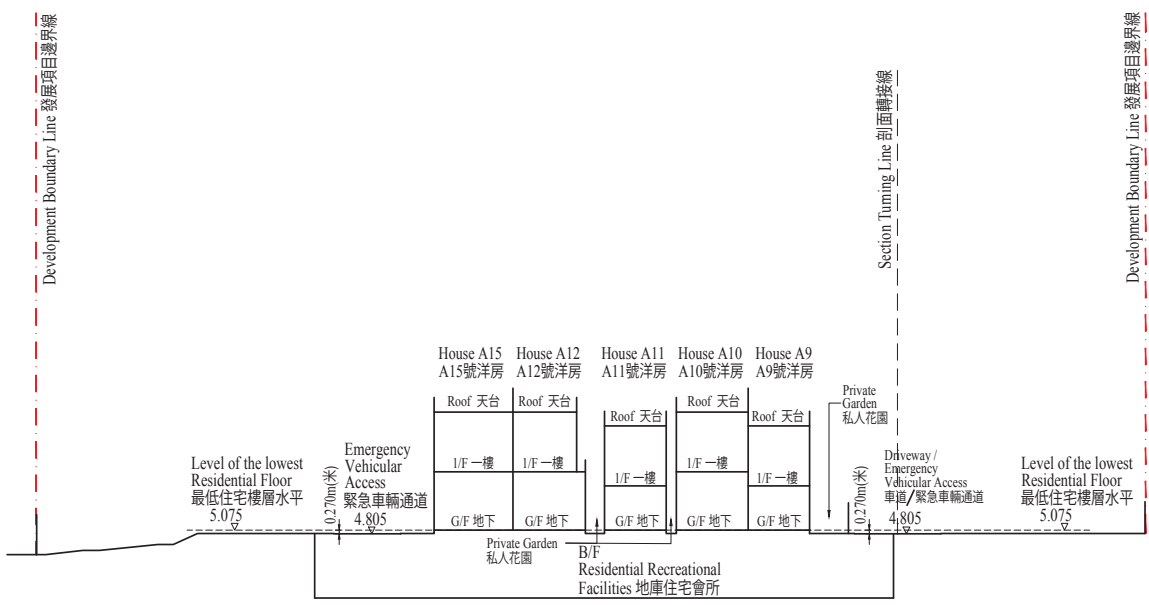
橫截面圖 M-M CROSS-SECTION PLAN M-M
