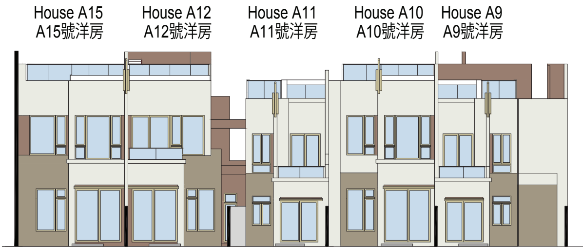
立面圖 34 ELEVATION PLAN 34
