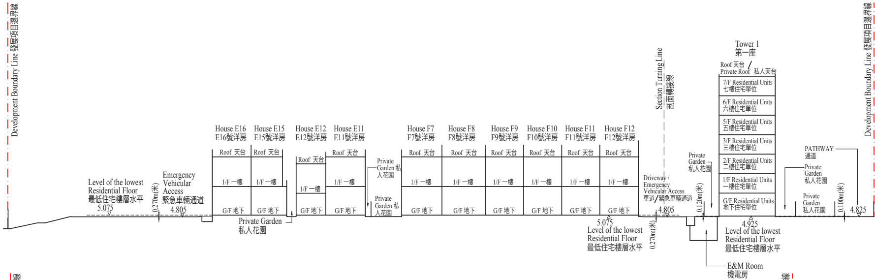
橫截面圖 E-E CROSS-SECTION PLAN E-E
